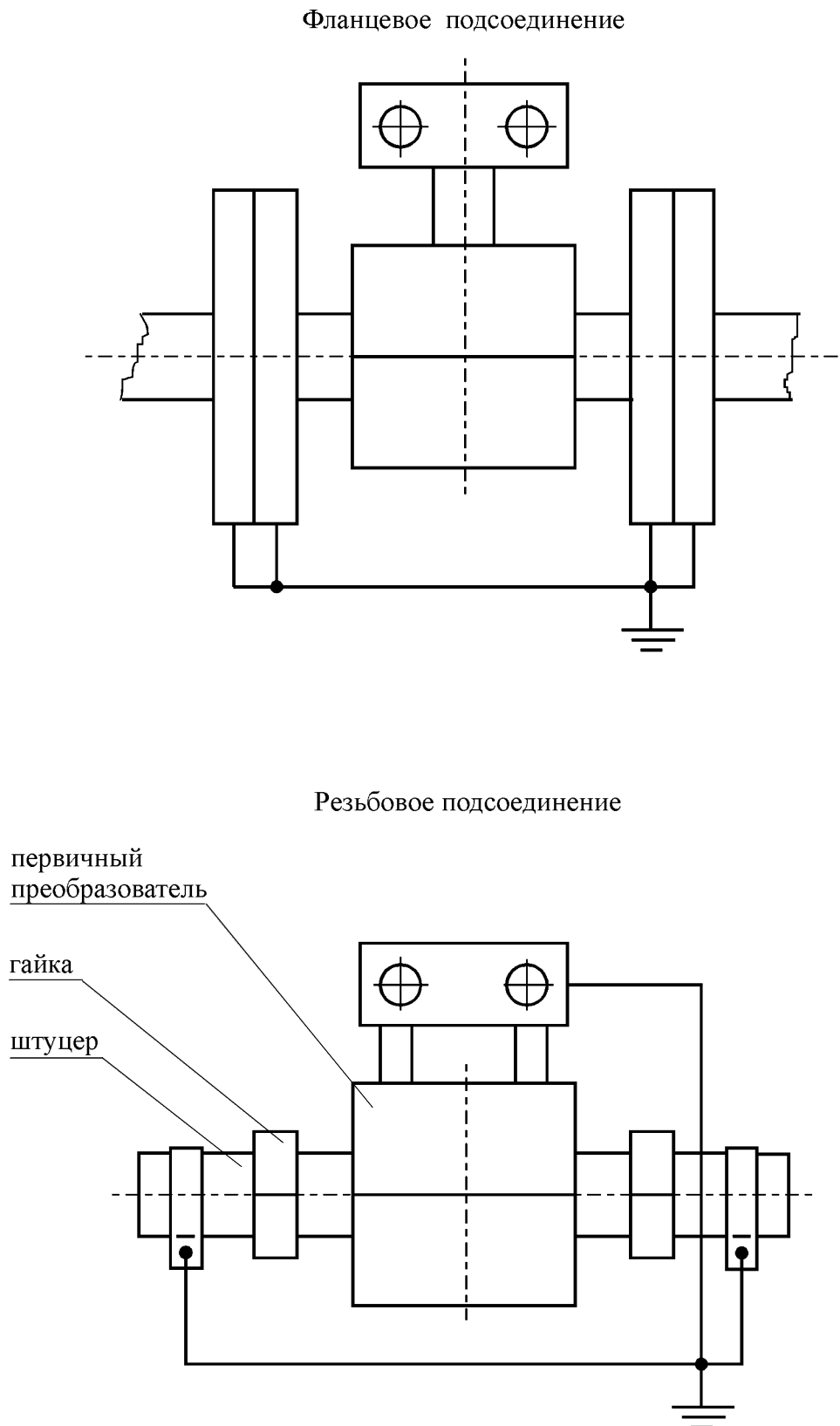
Рисунок 18 - Схема заземления первичных преобразователей
